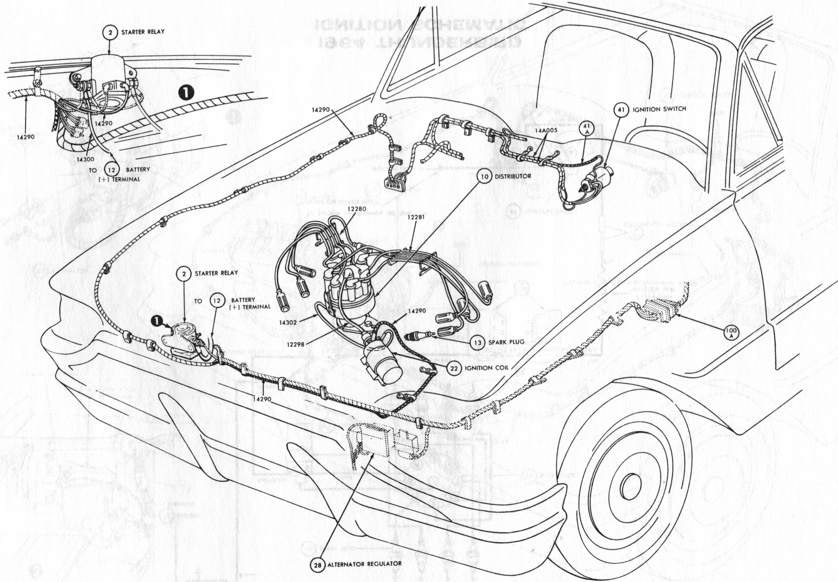
1964 THUNDERBIRD IGNITION WIRING
